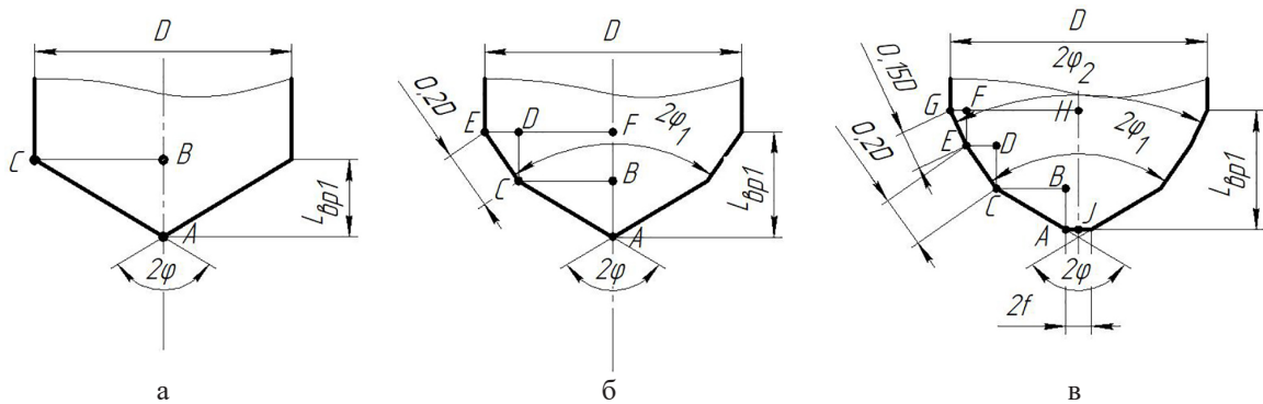
Рисунок 4 – Примеры расчетных схем для определения L_{сп1} некоторых видов сверл:
