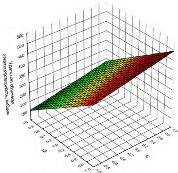
Рисунок 3 – Зависимость удельной объемной электропроводности раствора от входных факторов эксперимента
